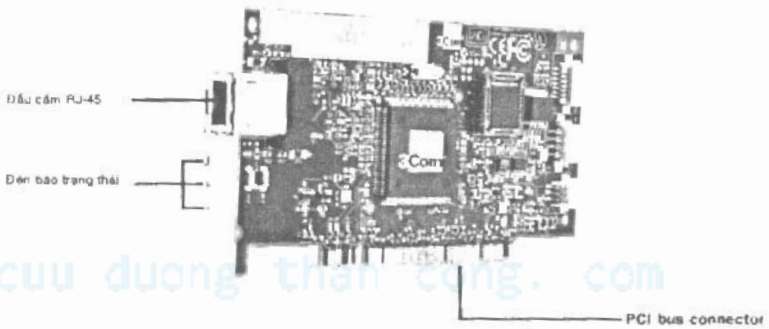
Hình 6.10 Card 3Com 3C905C-TX-M 10/100Base-T PCI Ethernet
