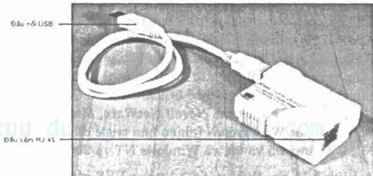
Hình 6.11 Card 3Com 3C460 Home Network USB Ethernet
