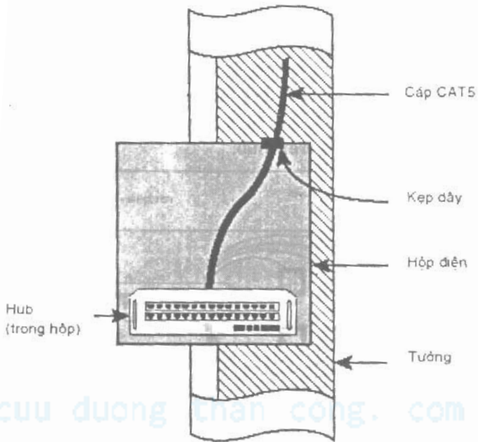
Hình 5.14 Hộp điện trên tường, đặt và đi dây cho hub.
