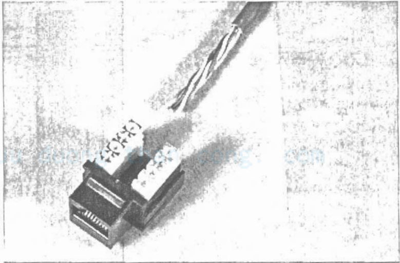
Hình 5.8 Chuẩn bị cáp CAT5 để nối vào đầu nối trong.
