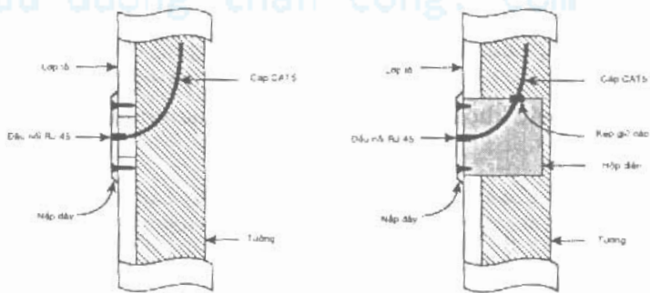
Hình 5.12 Gắn các ổ cắm lên tường.
