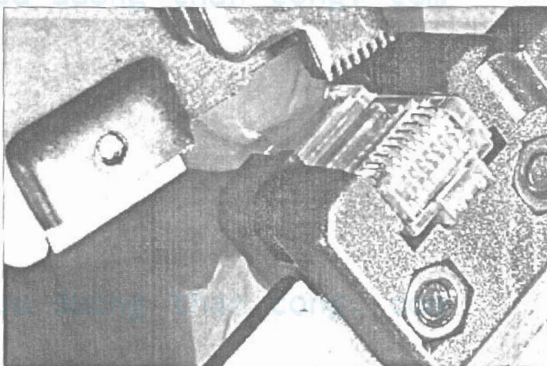
Hình 4.10 Bấm đầu cắm RJ-45
