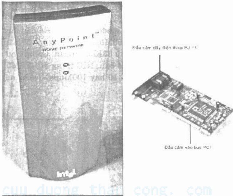
Hình 6.13 Card gắn ngoài và gắn trong
