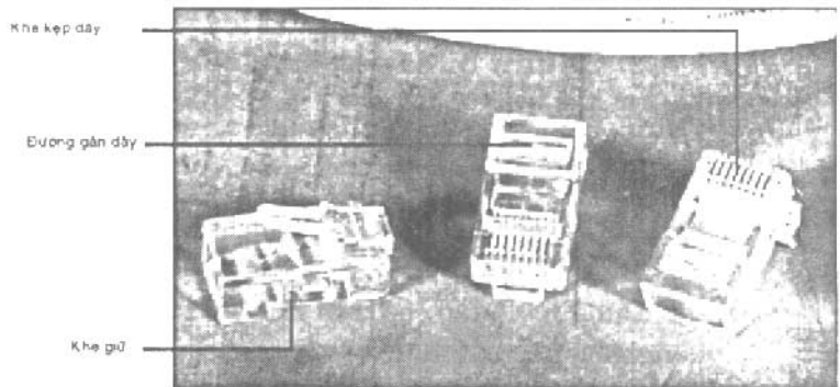
Hình 4.5 Đầu cắm RJ-45
