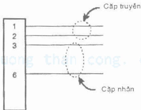
Hình 4.3 Dây cáp xoắn gắn vào các chân của đầu cắm RJ-45
