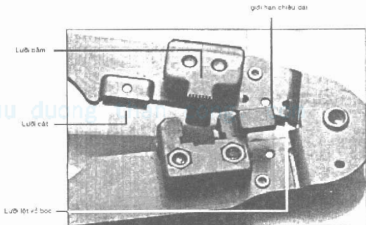
Hình 4.4 Kim bấm dây
