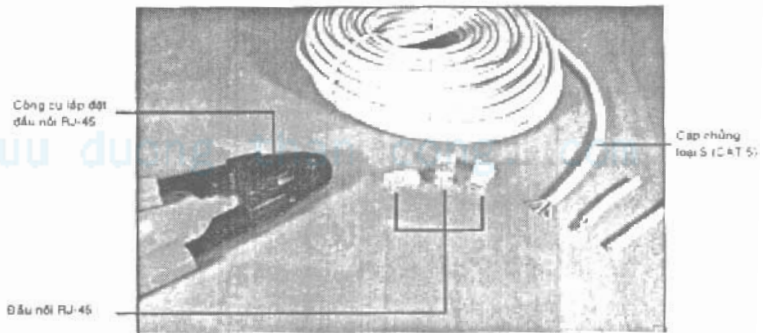
Hình 4.2 Dây cáp xoắn đôi và đầu cắm RJ45.
