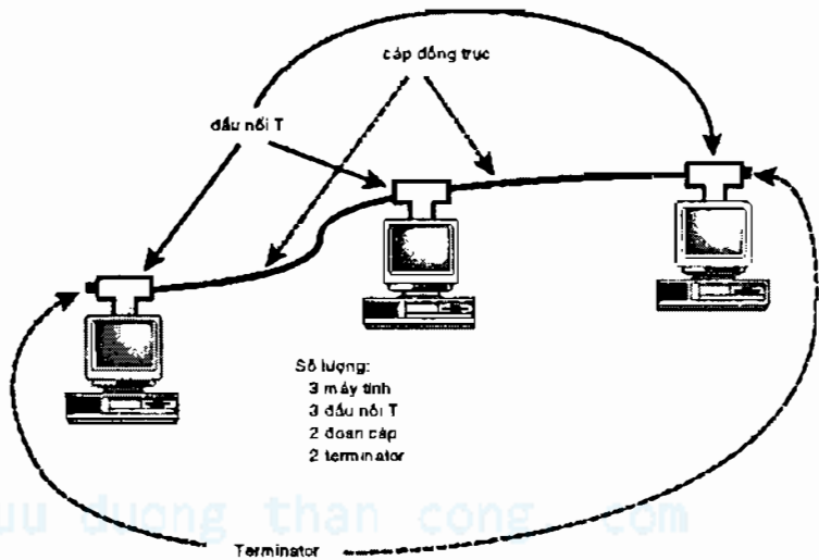
Hình 2.19 Các phần của một mạng 10Base-2
