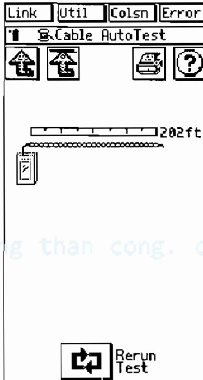
Hình 17.8 Đo chiều dài cáp.
