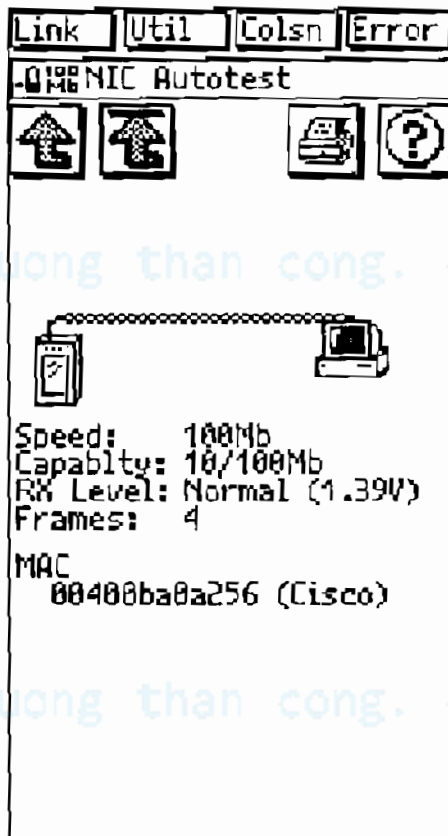
Hình 17.7 Kiểm tra card mạng của OneTouch.
