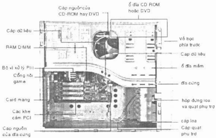
Hình 6.3 Phía bên trong của máy tính
