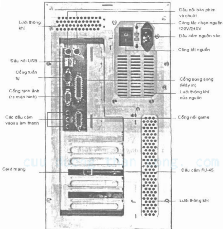
Hình 6.2 Phía sau máy tính
