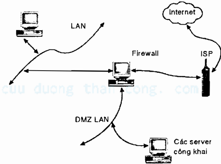
Hình 14.4 DMZ (Demilitarized zone) được sử dụng với firewall
