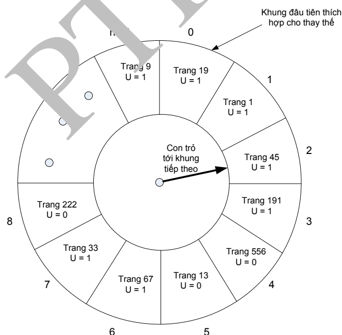
Hình 3.18 .Thuật toán đồng hồ
