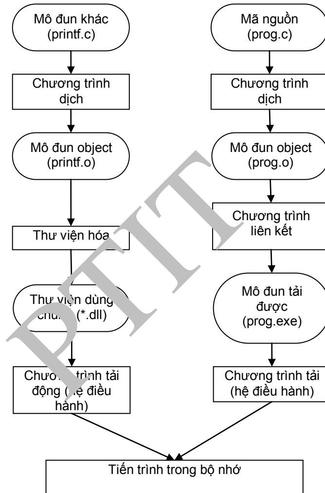
Hình 3.2: Liên kết động trong thời gian thực hiện
